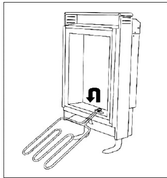
Figura 10 b - ACE 605
