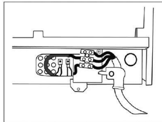
Figura 11 b - ACE 605
