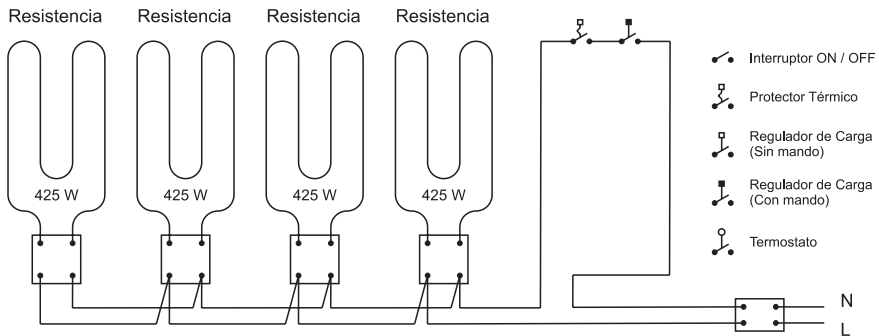
ACUMULADORES ACE-805, ACE-1205, ACE-1605
