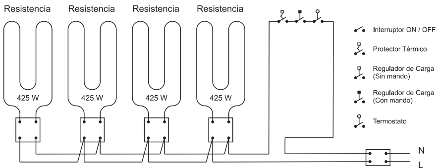
ACUMULADORES ACE-805 A, ACE-1205 A, ACE-1605 A
