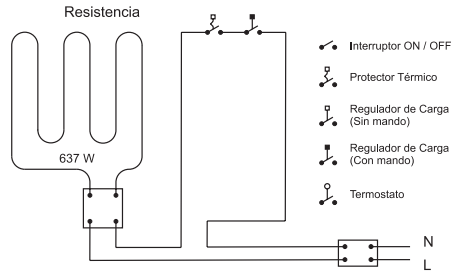
ACUMULADOR ACE-605
